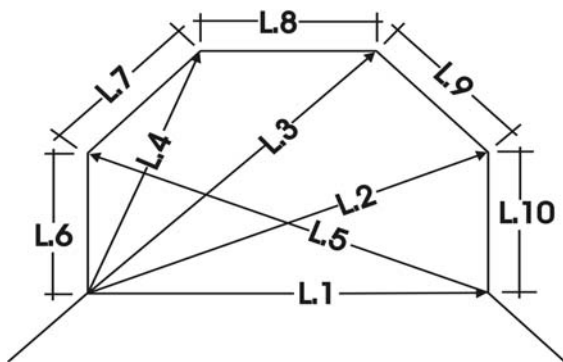
Optimale Erkervermessung
